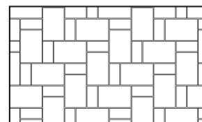
LEXA_P_AC_H2 Motif modulaire (25% A et 75% C)
