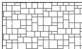
TRAFALGAR_P_ABCD_C2 Motif modulaire (85-90% ABC et 10-15% D)
