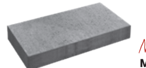
Module 60 60 x 305 x 600 mm 2 3/8 x 12 x 23 5/8 po
